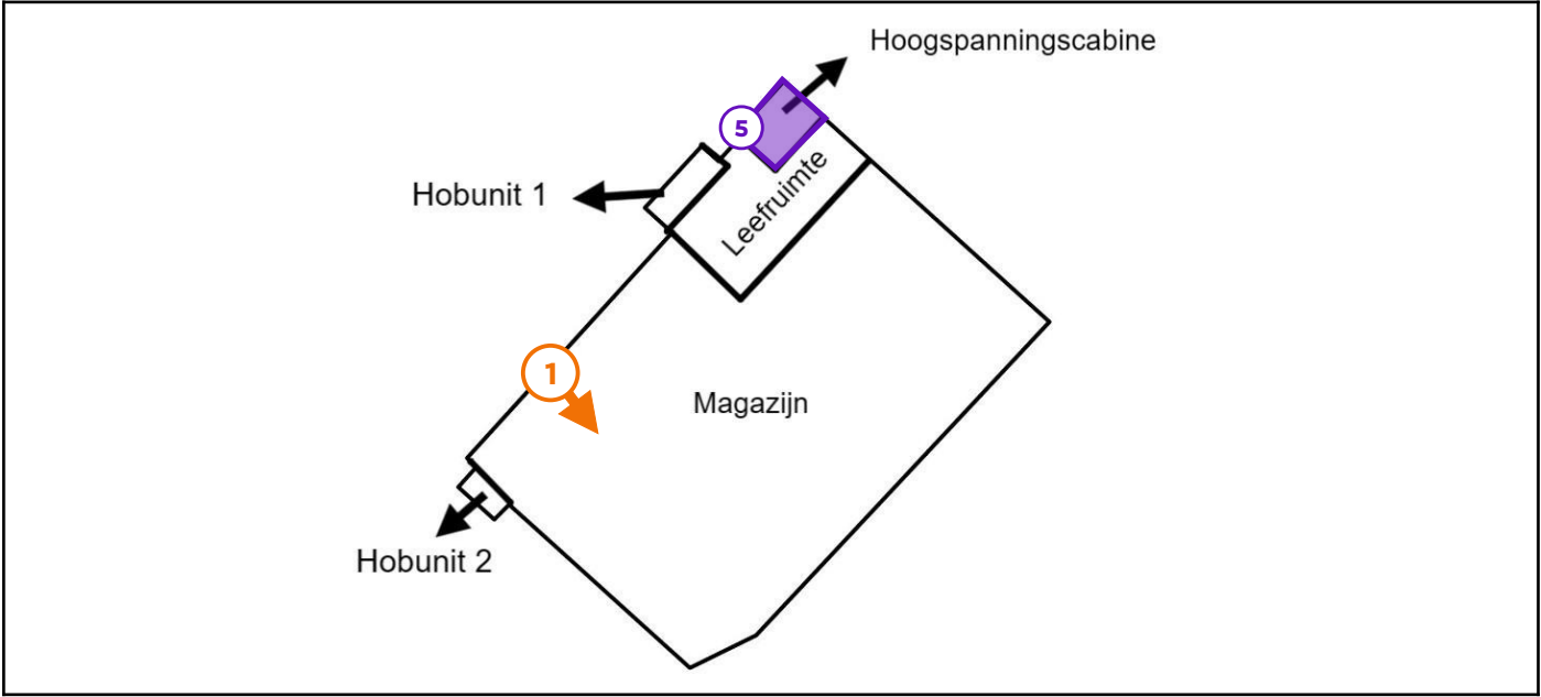
Legende van plan 1.3: Indelingsplan
